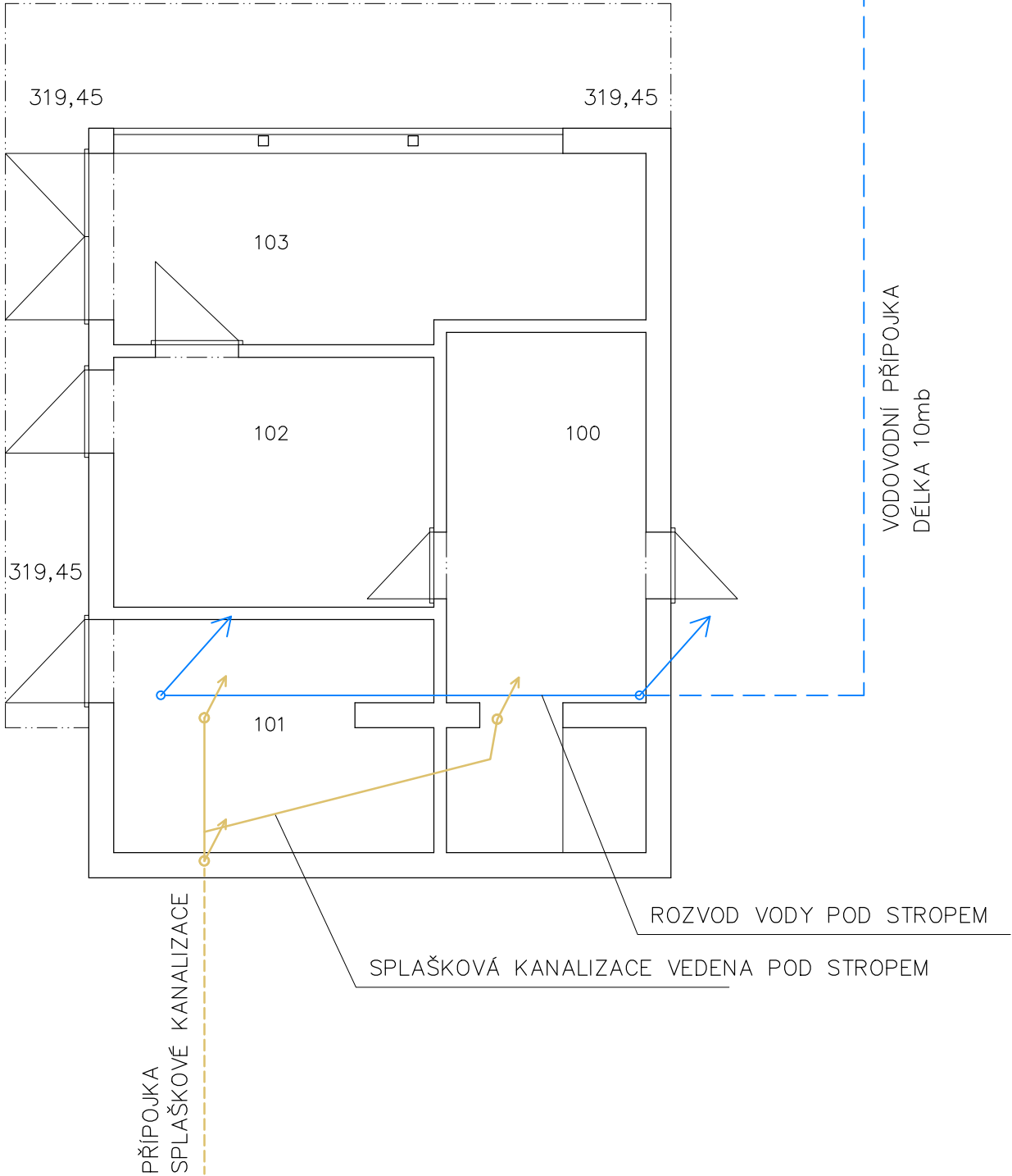
PŮDORYS 1.PP
