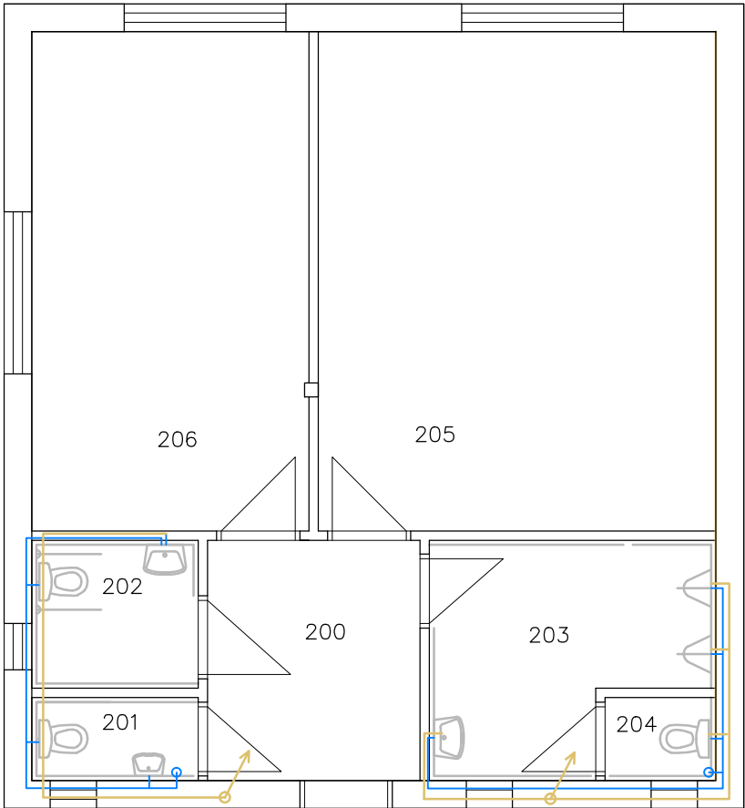
PŮDORYS 1.NP
