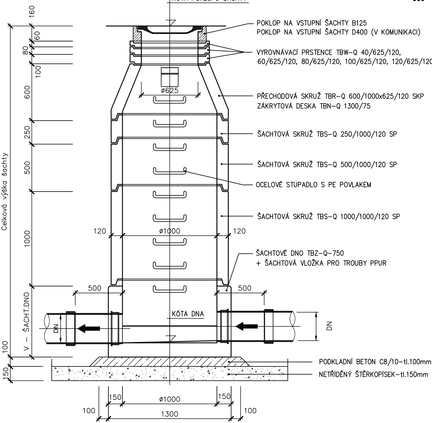
PODÉLNÝ ŘEZ
