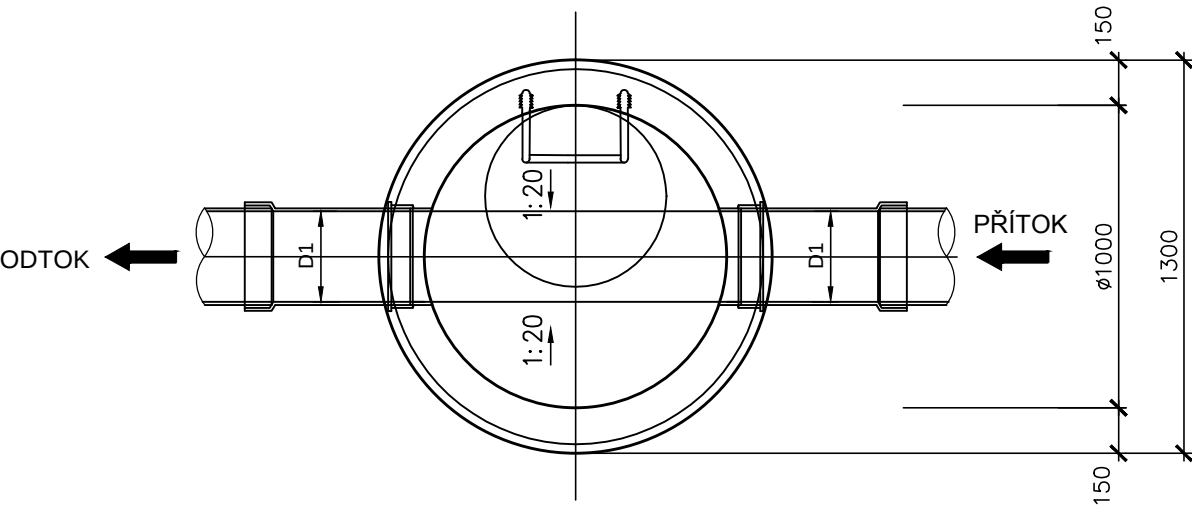
PŮDORYSNÝ ŘEZ V PŘÍMÉ
